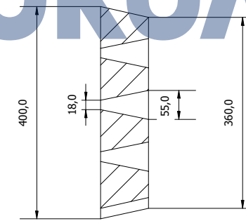
A-A ( 1 : 10 )
